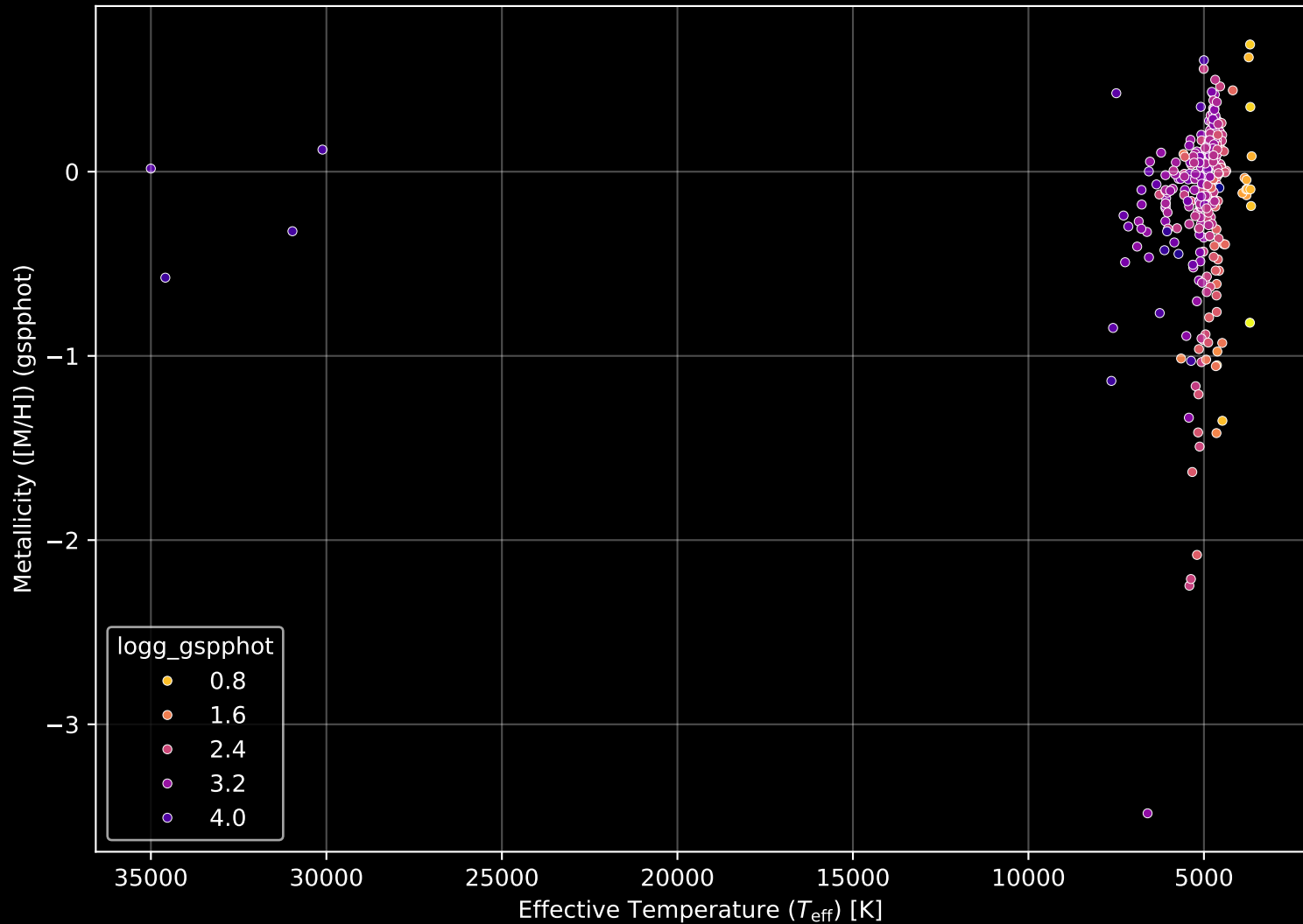
APOGEE DR17 Field: [005+08] Stellar Population Parameters (n= 348)
